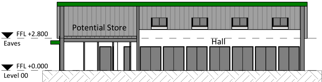
Section C-C 1 : 200
